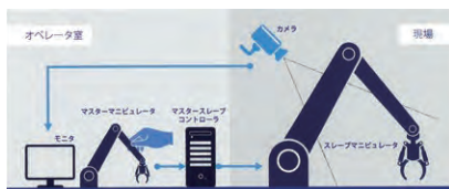
用途最適化テラーメード「マスタスレーブロボット」 Custom-made master / slave robots optimized for the application
