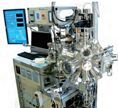
モバイルコンビレーザー MBE
