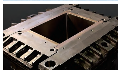
製鉄連続モールド（鉄の連続鑄造に野村のめっき・加工技術が使われています。） Continuous-casted iron mold (Nomura's plating and processing technology is used in continuous iron casting.)
